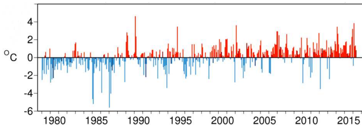
Slika 2. Odklon evropske povprečne mesečne temperature od povprečja obdobja 1981–2010, majski odkloni so obarvani temneje, vir: ERA-Interim
