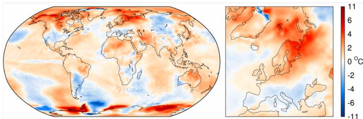
Slika 1. Odklon temperature maja 2016 od povprečja obdobja 1981–2010, vir: ERA-Interim
