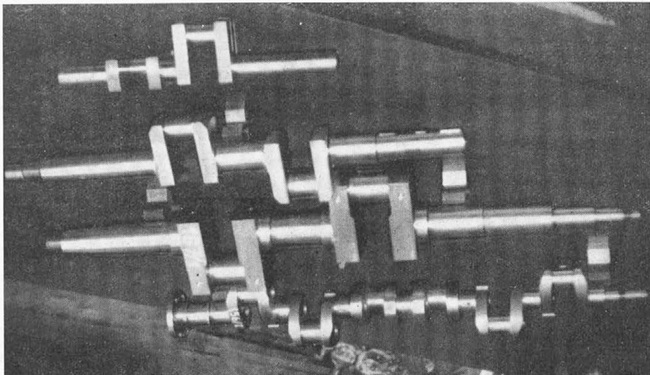
Kolenčaste osi — mojstrovina ravenskih fužin.
