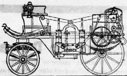
Brizgalnica kombinirana z motorjem
