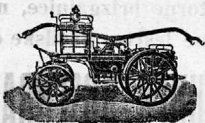
Predpisana četverokolna brizgalnica na peresih z enim ali dvema curkoma; močan pritisk vode
