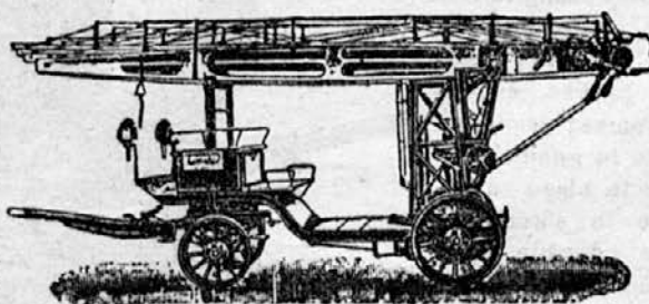
Mehanična sukalna lestva (rotačna lestva)
