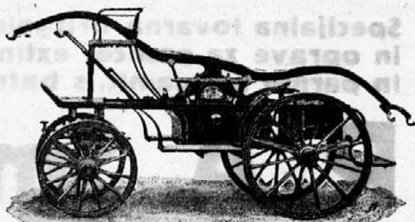
Četverokolna normalna brizgalnica.
