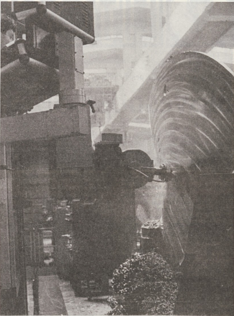
Tako pa stroj dela tisto, kar so donedavnega obdelovale človeške roke — hidravlične oblike lopate Kaplanovega gonilnika. (Foto: E. L.)
