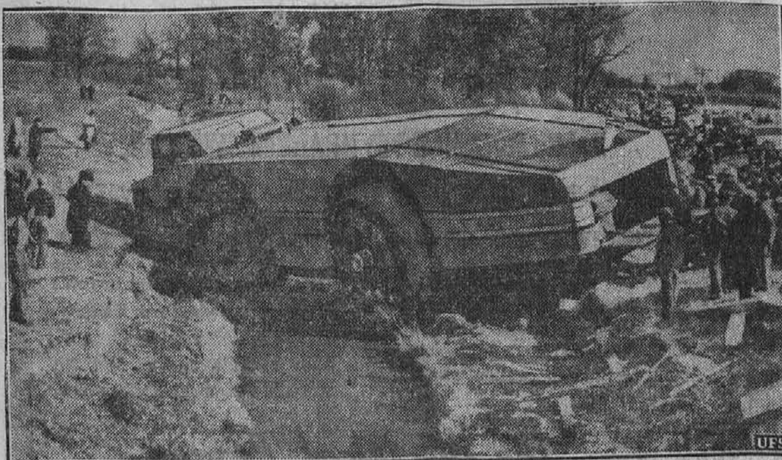
Ogromno vozilo, ki ga je vzel s seboj admiral Byrd na južni tečaj, da bo vozil ekspedicijo po tamošnjih snežnih pokrajinah. Slika kaže vozilo, ki je na potu iz Chicaga v Bostonu zašlo s poti v mal potok v bližini Gomer, Ohio. Vozilo je 55 čevljev dolgo, 15 čevljev široko in tehta 35 ton.
