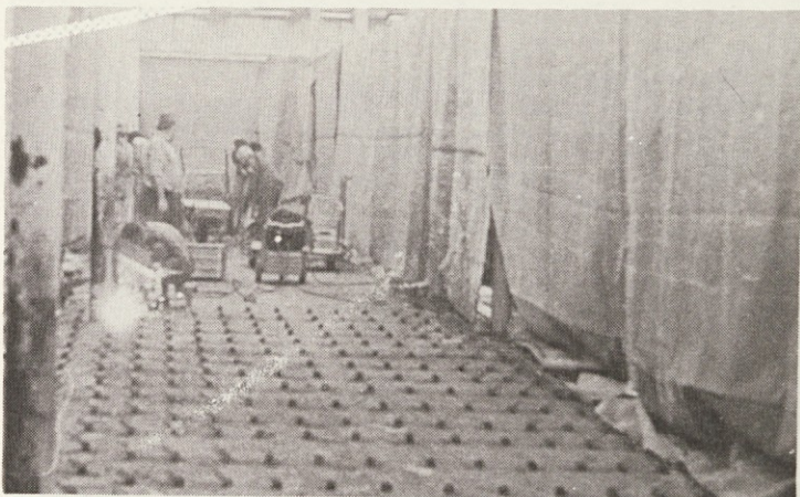
Varjenje armature temeljev za 15. in 16. predilni stroj Tekstima.
