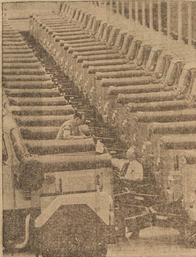
ZA TEŽAVNE OKOLISČINE — Slika kaže dve vrsti težkih tovarnjakov, izdelek White Motor Corporation tovarne v Kelowni v Britski Kolumbiji. Tovornjake bodo poslali v Aljasko, kjer jih bodo rabili pri gradnji oljevoda.
