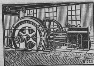
LANZOVE vročeparne Lokomobile z naravnost vezano Dynamom.
