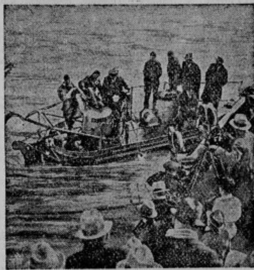
V Ameriki so se vršili pred kratkim poskusi s potapljačem, ki ga je inž. Simon Lake čisto svojevrstno skonstruiral. Potapljač se imenuje »Explorer«. Ima pa samo ta namen, da bo dvigal zaklade s potopljenih ladij. Potapljač je dolg samo 6 metrov in pol in točno 2 metra širok. Vzbudil pa je med inženjerji, oblastmi in znanstveniki veliko občudovanje. Oskrbljen je z zalogo stisnjene zrak, elektriko, telefonom in s pomožnim bolnom.
