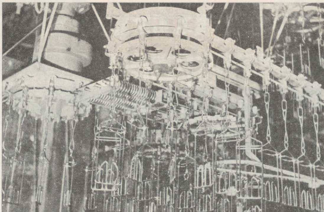
Pogonski mehanizmi in natezne naprave na novih tekočih trakovih v evisceraciji.
