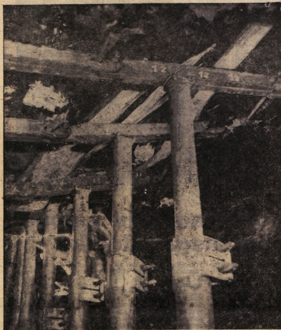
JEKLENE STOJKE »VALENT« IN JEKLENE STOPNICE Strojne tovarne Trbovlje v jami Trbovlje leta 1962
