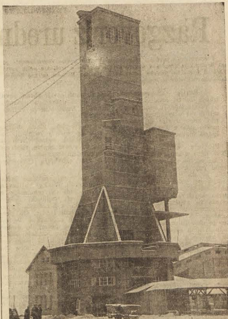
Novi, 43 m visoki izvozni stolp v Velenju, ki bo začel obratovati letos 31. decembra. Žične vrvi, ki jih je videti na sliki, vodijo do velikih bobnov v eni izmed najmodernejših strojin v Evropi
