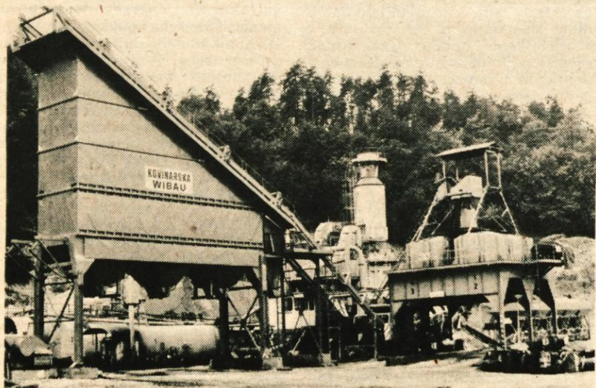
NOV TERMOSILOŠ V NAKLEM — Cestno podjetje iz Kranja je postavilo v asfaltni bazi v Naklem nov 400-tonski termosilos. Zaradi novega silosa se je proizvodnja v bazi povečala od nekdanjih 1000 ton asfaltne mase v šestnajstih urah na 1300 ton. V novem termosilosu asfaltna masa lahko počaka naslednjega dne, saj se ohladi le za eno stopinjo na uro. (jk) — Foto: F. Perdan
