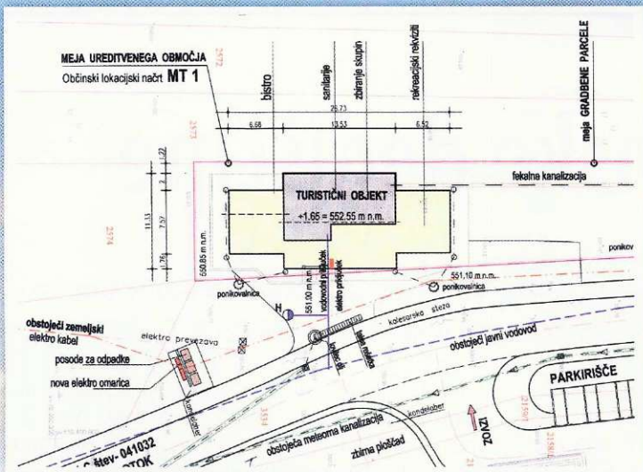
Načrt vstopne točke na Cerknško jezero
