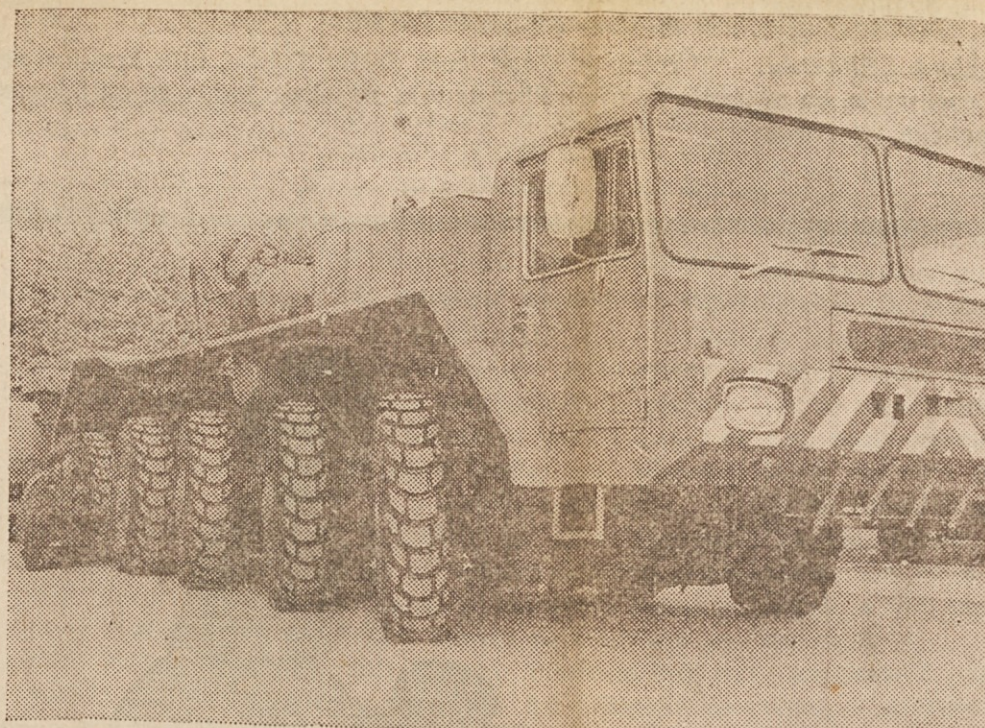
ZA IZREDEN TOVOR — Na sliki vidimo tovornjak s 16 kolesi na petih premakljivih oseh spredaj in na treh zadaj. Tovornjak je težak 96 ton in ima motorje s skupno 530 konjskih sil. Prevaža žerjav, ki je sposoben dvigniti 400 ton. Slika je bila posneta v Lau- fu na Nemškem.
