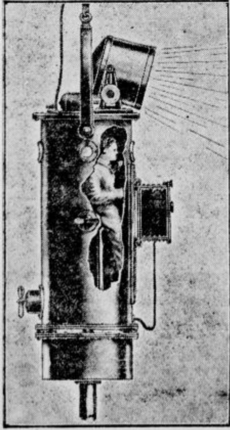
Morska patrona za potapljače. S pomočjo tega aparata, v katerem je prostora za dva moža, so mogoča raziskovanja v takih morskih globinah, ki so bile doslej nepristupne. Patrona je opremljena z močno električno lučjo, telefonom in filmskim aparatom. Kisik za dihanje se proizvaja v patroni.
