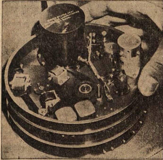
Registrator kozmičnih žarkov, ki so ga vdelali v drugi ameriški umetni satelit
