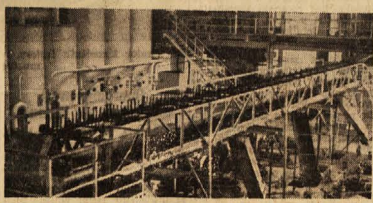
V Županji smo zgradili po vojni novo moderno tovarno sladkorja. V tej tovarni je ves delovni pos postopek mehaniziran.
