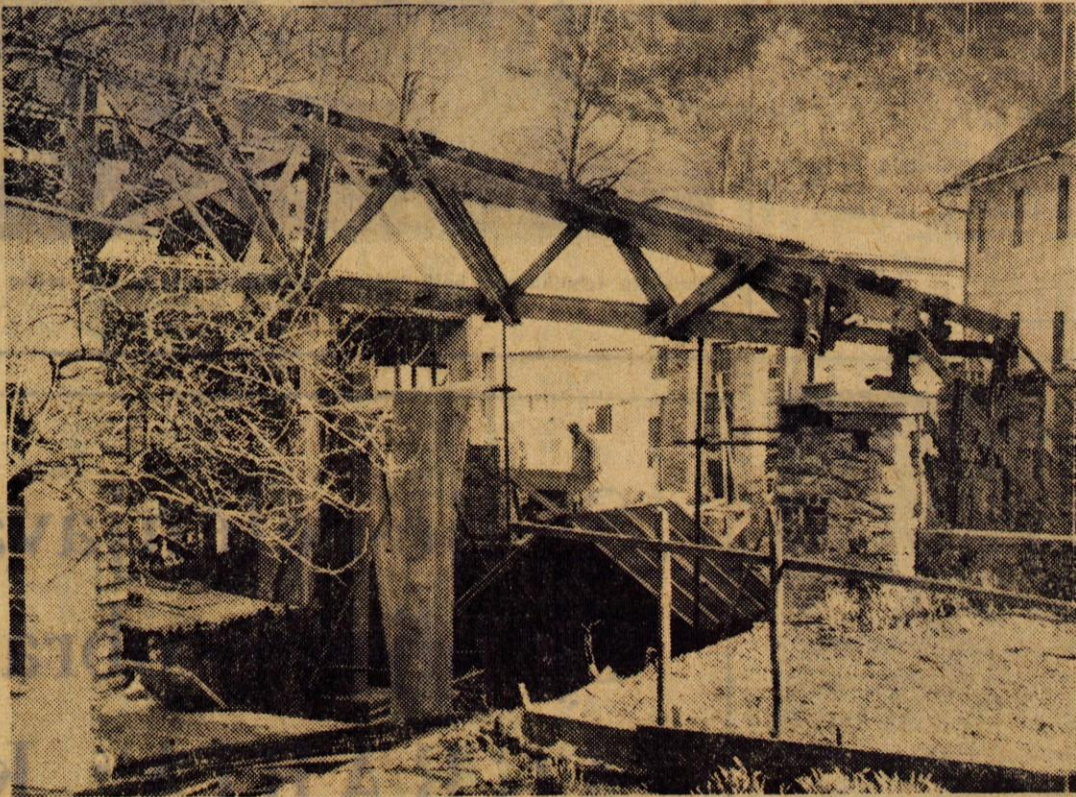
Tržiška tovarna kos in srpov bo v kratkem zaključila z gradnjo novih prostorov, v katere bo lahko preselila sedanji obrat, ki je na prostoru, kjer bodo začeli z gradnjo stanovanjske stolpnice. — Na sliki: razširitev delavnice za ročno orodje
