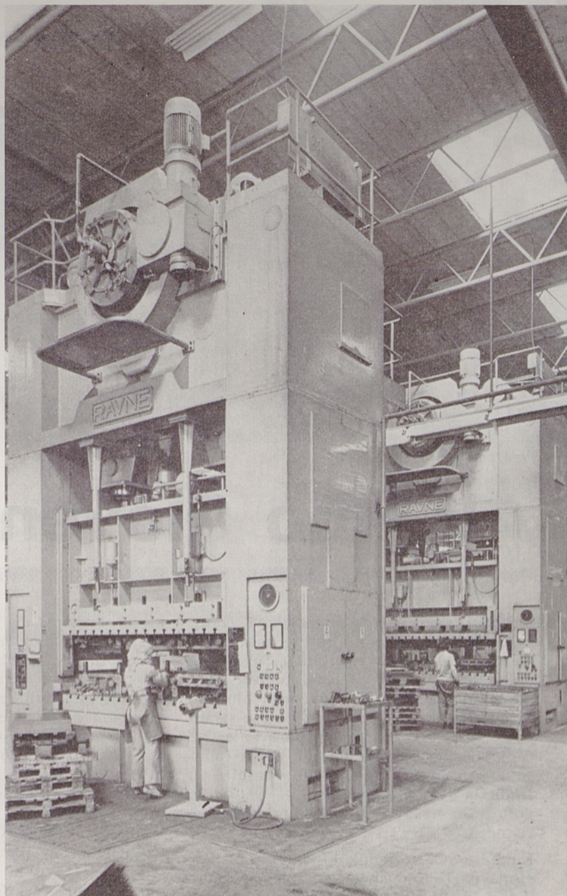
Velika stiskalnica za oblikovanje pločevine v tovarni »Gorenje«
