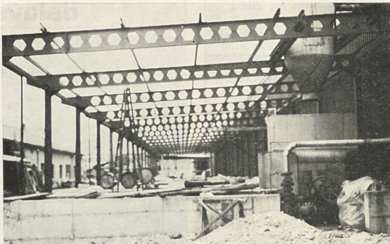
Jeklena konstrukcija montažnega prizidka pri petem papirnem stroju; desno je nov razpuščevalce izmeta za V. PS
