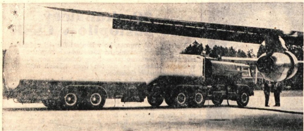
Petrol iz Ljubljane je za potrebe letališča na Brniku v Italiji kupil ogromno avtocisterno za letalsko gorivo, ki jo bodo uporabljali ob pristankih velikih letal. V sredo so jo prvič uporabili. Cisterna sprejme 40.000 litrov goriva, veljala pa je 50 milijonov starih dinarjev. To je vsekakor velika pridobitev za letališče. — (jk) Foto: F. Perdan
