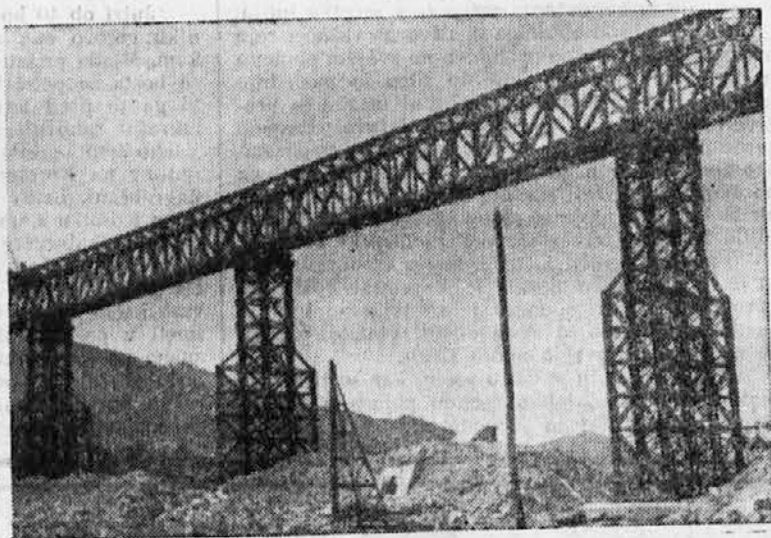
Due fotografie del viadotto di Borovnica polse a 80 giorni di distanza. — Sliki borovniškega mostu, narejeni komaj 80 dni druga za drugo.
