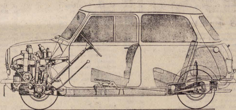
V tej shemi vidimo vso domiselnost Isigonisovega projekta prvega minija.
