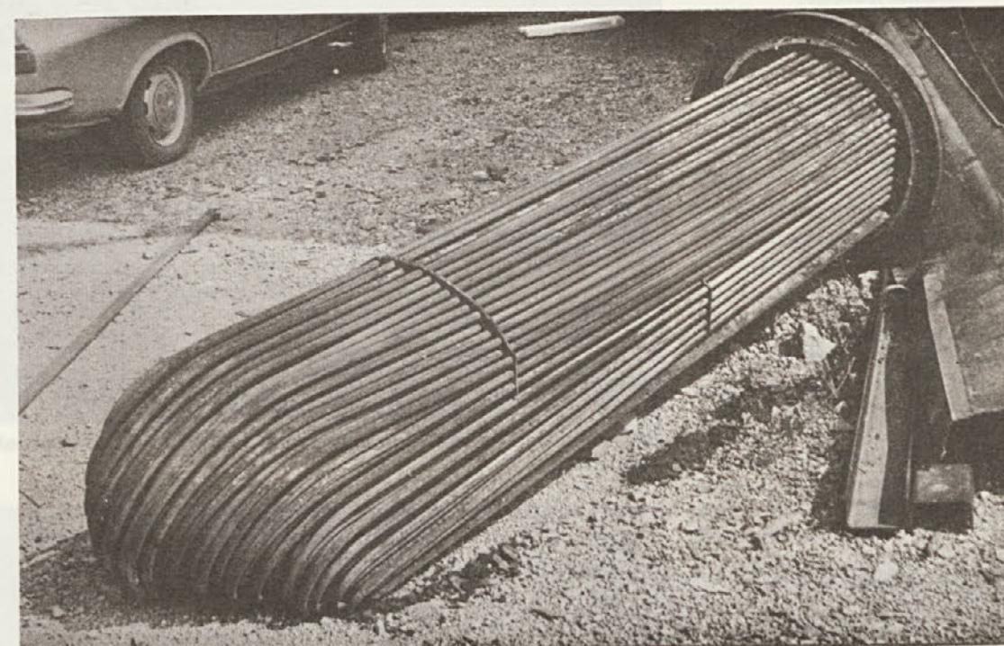
Tako je izgledal grelec, ki smo ga zamenjali. Kar 900 kg bakrenih cevi je v njem
