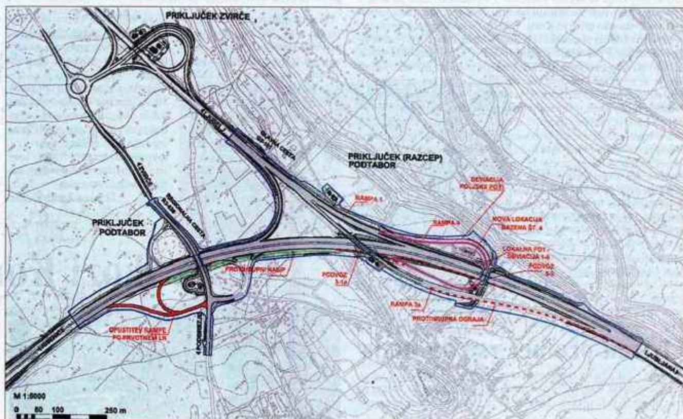
Na desni strani skice je z vijolično barvo označena nova, četrta rampa.
