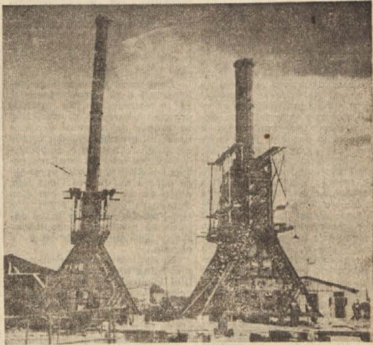
Montiranje novih destilacijskih naprav v rafinerijah v Sisku
