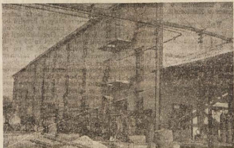
Oddelek za izdelavo monoklorbenzola in solne kisline
