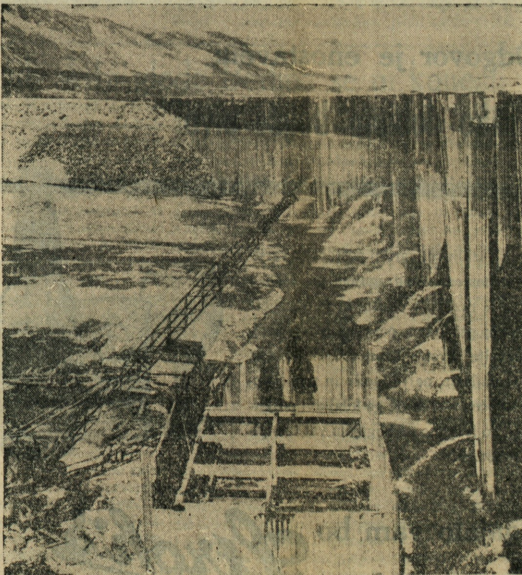
ZARADI VARNOSTI — V jekleni steni zapore, ki omogoča gradnjo John Day jezusa v južnem delu srednjega Washingtona, je vrsta lukenj, skozi katere teče voda. Vodni curki, ki jih vidimo na sliki, zmanjšujejo pritisk za jekleno steno zbrane vode.
