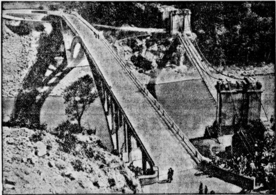
Novi most med Indijo in Tibetom. Indijo in Tibet loči dolina Terta. Čez njo je doslej vodil viseči most (na desni), ki je bil že star. Sedaj so zgradili nov moderen most (na levi).
