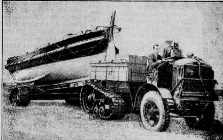
Angleži so izvršili uspele poizkuse dovažanja obrežnih rešilnih motornih čolnov na kraj nesreče s traktorji.
