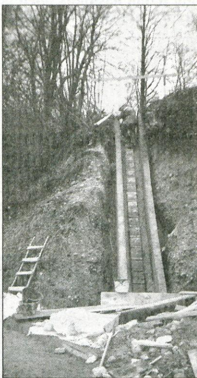
Izgradnja kanalizacijskega kolektorja iz Pristave se končuje, odplake pa bodo končale v Tržiški Bistrici.
