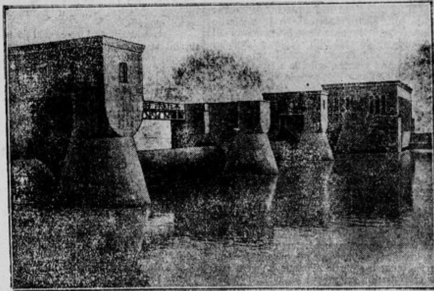
Vodne zgradbe ob Ruhri. Nemci so zgradili ob reki Ruhri ogromen valjni jez, ki zadržuje vodo v jezeru, obsegajočem tri milijone kubčnih metrov, da se tamkaj izčisti. Jez more odvajati 2400 kubčnih metrov vode na sekundo in služi obenem za izrabo vodne sile in svrhu proizvodnje elektrike. Na uro se proizvaja 48.000 kilovatih ur. Stroški za zgradbo jezusa znašajo 7 milijonov mark.
