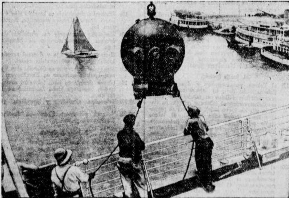
Amerikane William Beebe se v svoji krogli spušča v morské globine. Krogla je spodaj močno obtežena s kovinskimi ploščami, da pade — ko se spuščalna vrv odklopi — čim globlje v morje. Na morskem dnu pa se te plošče odklopijo in krogla se sam s pomočjo zraka, ki je v njej, dvigne na površje. V tej krogli se je W. Beebe spustil 900 m globoko. Namenjena je le raziskovanju velikih morských globin.
