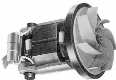
Sesalna enota 319.3.000 (Uy 66 40 A 10/13) za vgradnjo v sesalnik [5].
