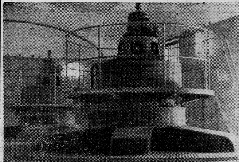
V novi hidroelektrarni Moste se poltuzsko obratujeta prva dva agregata po 5000 kilovatom. Hidroelektrarna bo v kratkem slovesno izročena svojem namenu. Na sliki vidimo oba generatorja v zgornji dvorani, pod njima pa sta v spodnji dvorani obe turbini, izdelani v Litostrju.
