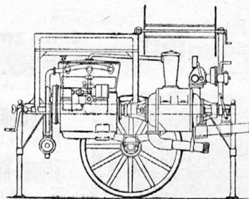
Motorna dvokolna brizgalnica z batnim brzotekim črpalom za visoki pritisk
