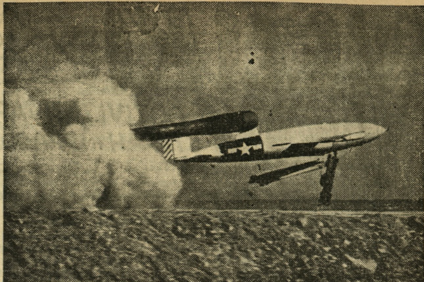
Raketno letalo na poletu
