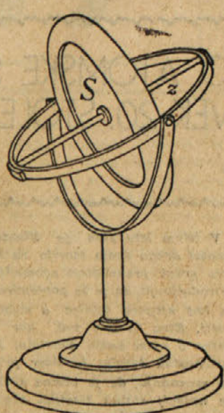
Do ladijskih stabilizatorjev so prišli s pomočjo dognanj te preproste naprave, ki jo imenujemo girokop. Njegova bistvena dela sta masivno in homogena kolo «S», ki je s pomočjo kardanskega ustroja priključeno na pravokotno os «Z».
