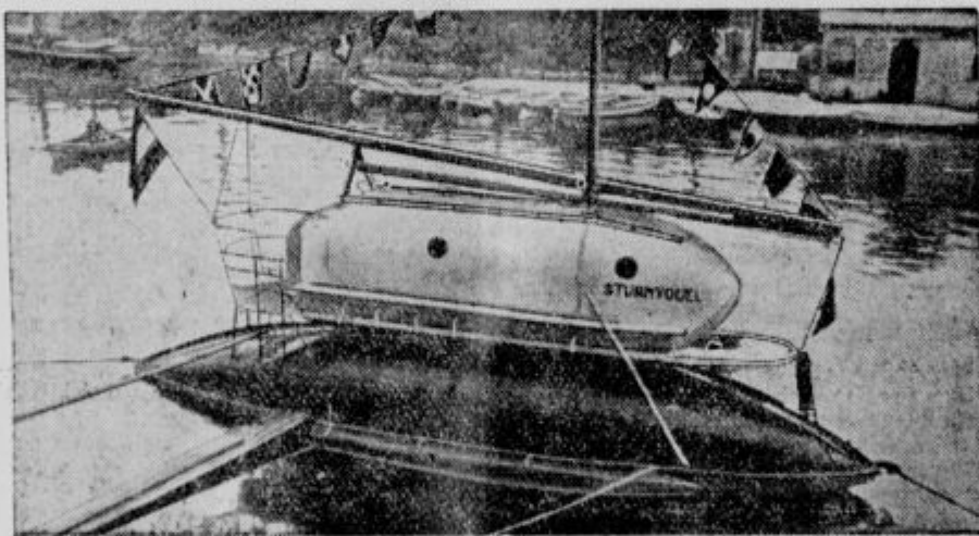
Nova nepotopljiva ladja »Sturmvoegel«, ki se odpravlja iz Rotterdama na pot okrog sveta. Ladja je dolga 9 metrov; pod njo se nahaja skladišče, ki se da povečati za 4 metre v globino. Obtežitev pod ladjo preprečuje, da se čoln ne more prevrtniti. Poleg jader ima ladja tudi pomožni motor 10 k. s.
