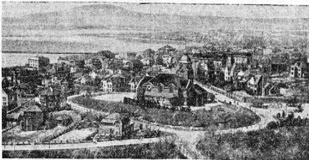
Kitajsko mesto Tsingtan, ki so ga Kitajci sami zažgali, da ne bi bilo kot obrežno mesto Japoncem v preveliko oporišče.
