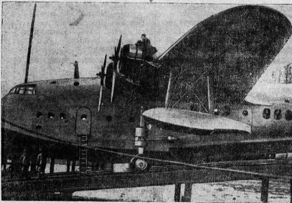
V Rochesteru v Angliji se gradijo za angleško zračno službo nova orjaška letala, ki dosežajo na uro preko 350 km. Ta letala so zgrajena tako, da ležijo posamezne kabine d ruga nad drugo.
