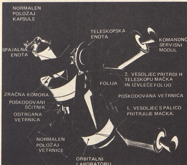
Skica enega izmed reševalnih načrtov: pritrjevanje zasilne folije nad razgaljenim delom Skylabovega trupa.
