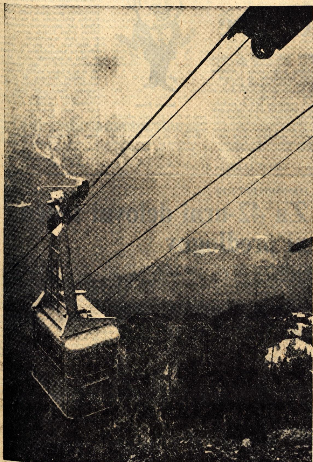
Za praznik dela bodo v Bohinju izročili namenu 1500 metrov dolgo žičnico z dvema gondolama, v katerih bo prostora za po 20 ljudi. Škofjeloški Transurist se je gradnje tega objekta lotil pred tremi leti in ga bo investicija veljala 280 milijonov dinarjev. (Reportaža o žičnici na Vogel berite na zadnji strani)
