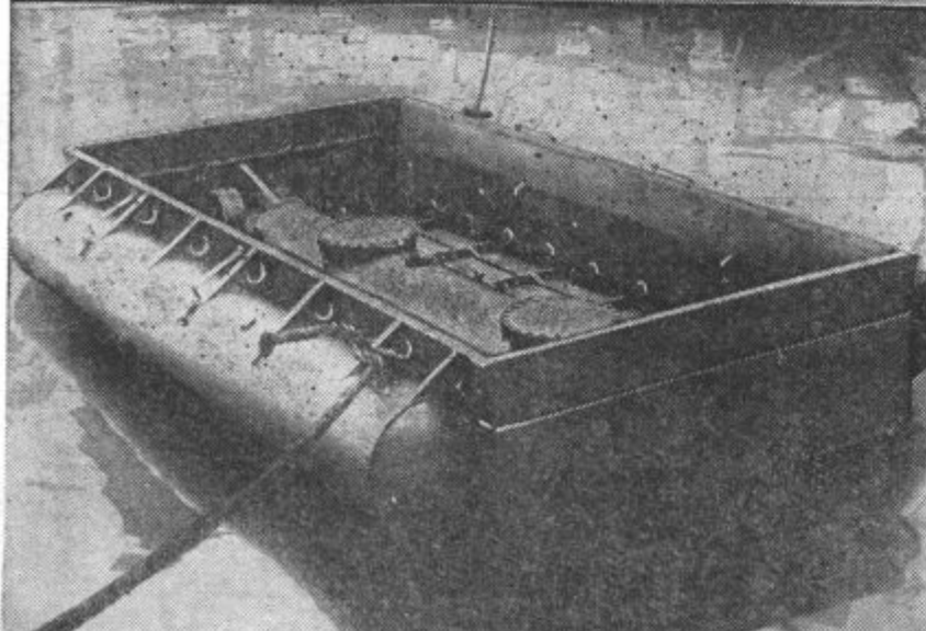
NOV NAČIN ZA RESEVANJE PODMORNISKIH POSADK. Podmorniške katastrofe zadnjega časa so dale tudi italijanskim strokovnjakom pobudo za gradnjo priprav, ki naj bi rabile kot reševalne priprave v takšnih primerih. Tako preizkušajo ta čas neko vrsto splava, ki se pritrdi na podmornico in ga je mogoče ločiti od nje s pripravo v njeni notranjosti. Splav se dvigne potem na površino morja, s seboj pa nosi do 40 mož posadke. Slika nam kaže z mornarji natovorjeni splav, spodaj pa je prazen. Valj v njegovi sredini vsebuje motor, radijski aparat in živež
