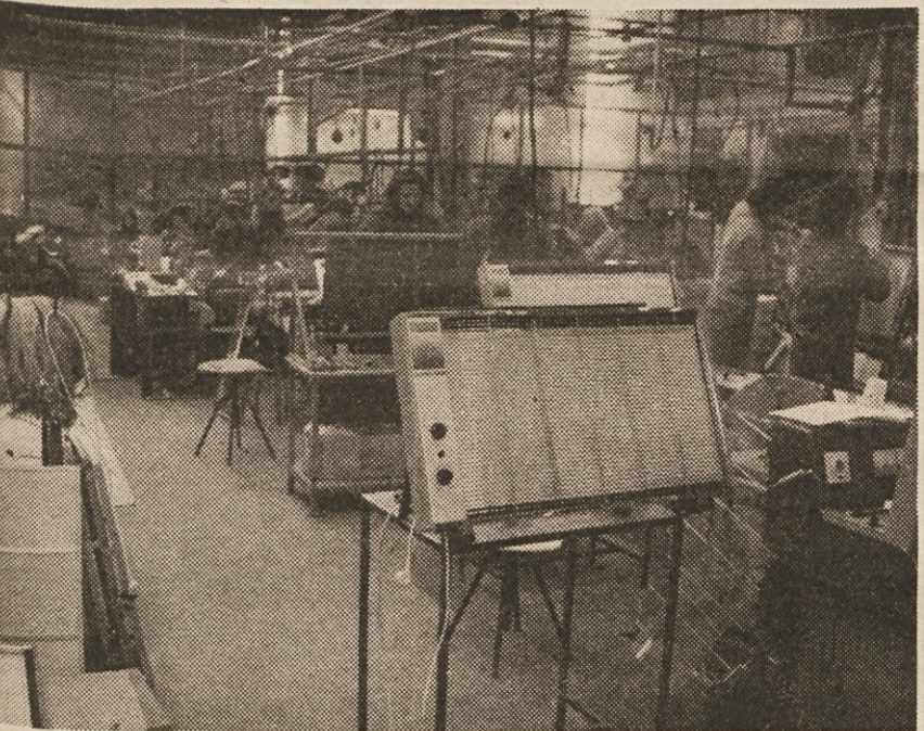
Montažni trak modulnih peči v TOZD TGA.
