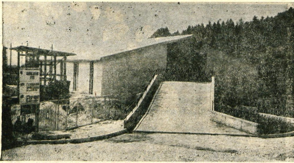
Splošno gradbeno podjetje Projekt iz Kranja je zgradilo v novem stanovanjskem naselju na Bistrici pri Trzinu garažo. Prvi objekt ki ga prikazuje naša fotografija, je že zgrajen. V njem je prostora za 60 avtomobilov. Ena garaža stane 13.000 dinarjev. Projekt namerava zgraditi še dva podobna objekta takoj, ko bo za nove garaže dovolj zanimanja. (jk) — Foto: F. Perdan
