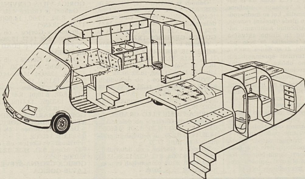
Prerez notranjosti bivalnega avtomobila.
