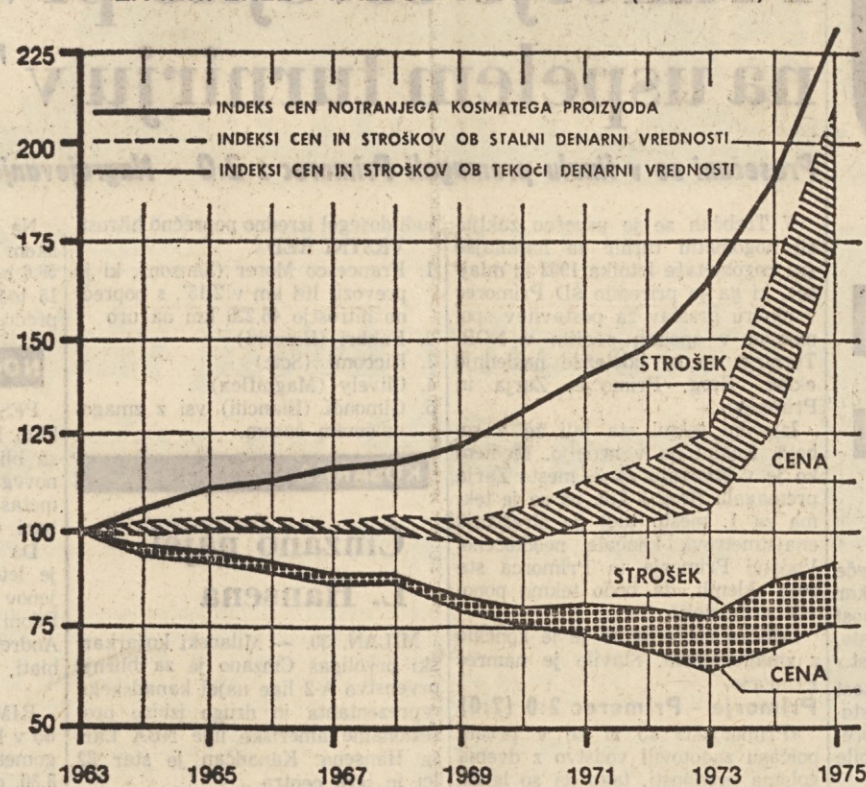
PRIMERJAVA MED INDEKSI SREDNJE CENE IN STROŠKA ZA kWh ENEL V RAZDOBJU 1963-1975 - (1963 = 100)
