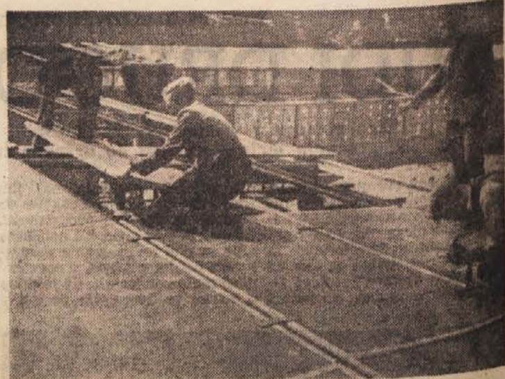
Stramit je zelo primeren tudi za izdelavo nadstrešij. Seveda je takšno streho spričo vremenskih razmer vseeno potrebna prekritja še s strešno lepenco, s ploščevino ali s čim podobnim
