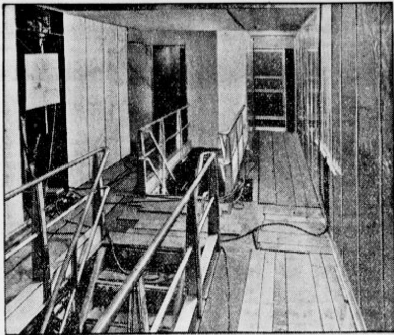
Leteči hotel. Na sliki vidimo stopnišče v nemškem zrakoplovu »LZ 129«, ki ga sedaj grade. Sredi decembra bo ta orjaška ladja opravila prvi poskusni polet. Dolga je 28 metrov ter v prerezu 41 metrov široka.
