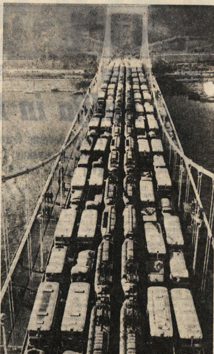
Uspehi tehnike: Elizabethin most v Budimpešti je zelo »eleganten«, na prvi pogled bi se zdel kar šibak, ker je v glavnem iz železa in jekla in ne iz kamna. In vendar zmoro ogromno breme. Na sliki vidimo kolodirane mostu, ko so za preizkušnjo speljali nanj kar 2000 ton tramvajev, avtobusov in drugih vozil, ki v šestih kolonah počasi drsijo čez enega brega na drugega.
